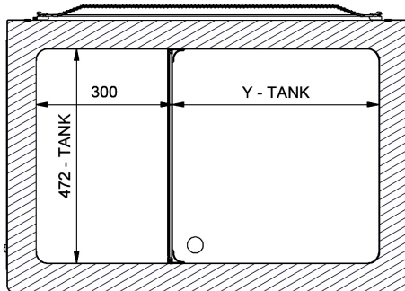
B-B ( 1/10 )
