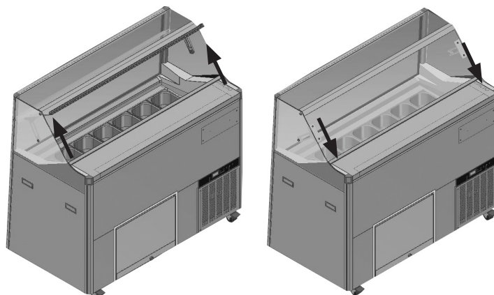
APPARECCHIO APERTO
